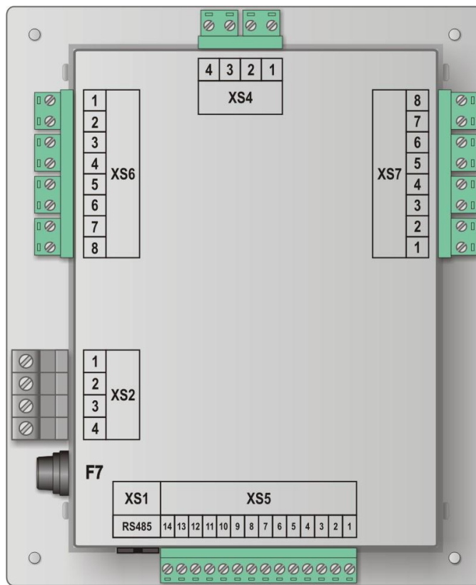
Рис 6.1. Клеммы и разъёмы подключения контролера (вид сзади).
