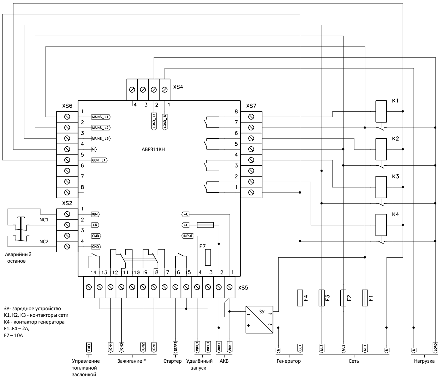
Рис 6.2. Пример схемы подключения контроллера ABP311KH.
