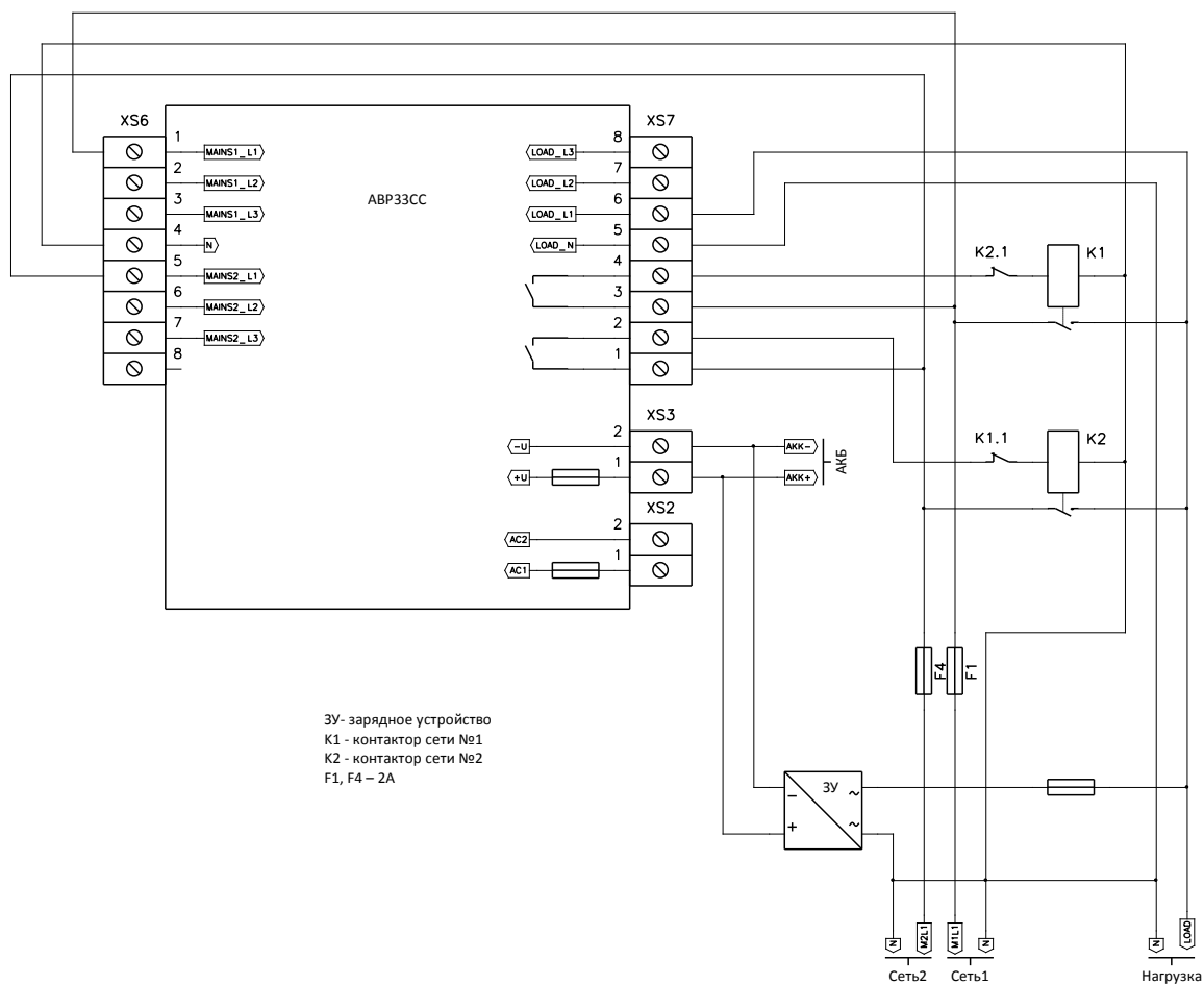
Рис 6.5. Пример схемы однофазного подключения контроллера АВР33СС с подключением внешнего зарядного устройства.
